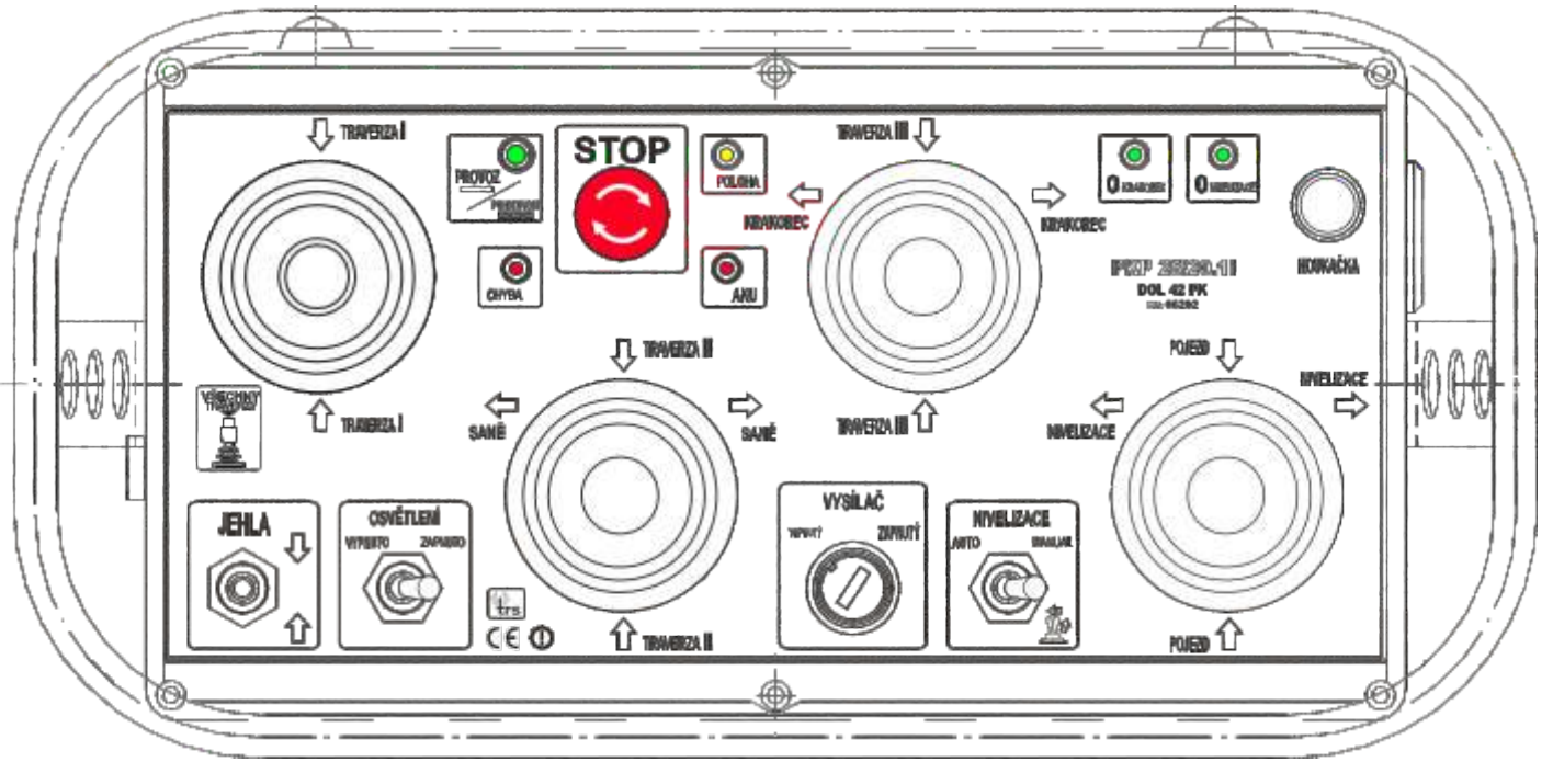
Pokladač kolejových polí PKP 25/20
